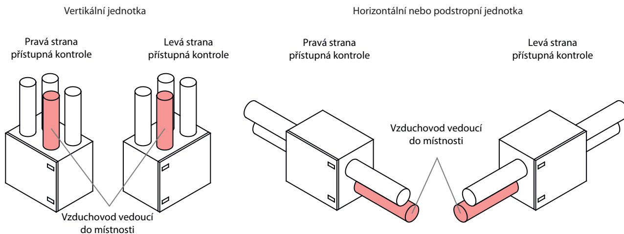
Obr. 2. Klasifikace jednotek podle strany přístupné kontrole
