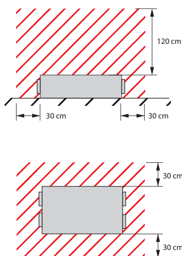
Obr. 5. Minimální prostor potřebný pro údržbu
