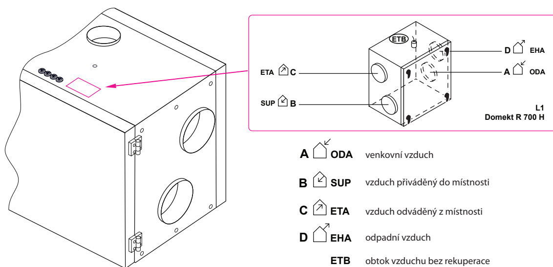
Obr. 8. Označení vzduchovodů
